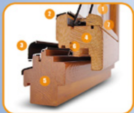
Przekrój przez okno (widok od wewnątrz)
